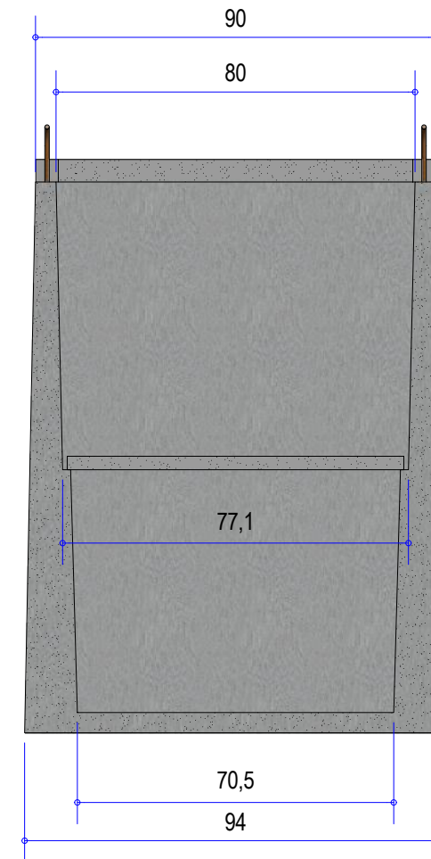
DOORSNEDE B-B COUPE B-B
